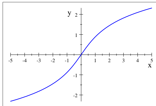
Funktion \ln(x + \sqrt{x^2 + 1})
