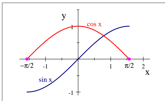
Die Graphen von \cos x und \sin x (rot) auf [-\frac{\pi}{2}, \frac{\pi}{2}]
