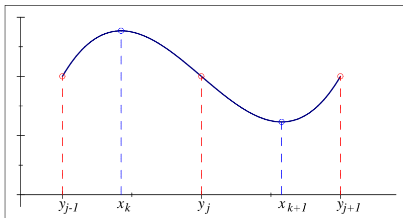
Lokale Extremumstellen x_k, x_{k+1} und ein Wendepunkt y_j
