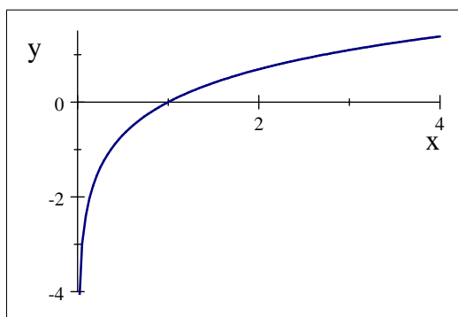
\ln x ist konkav
