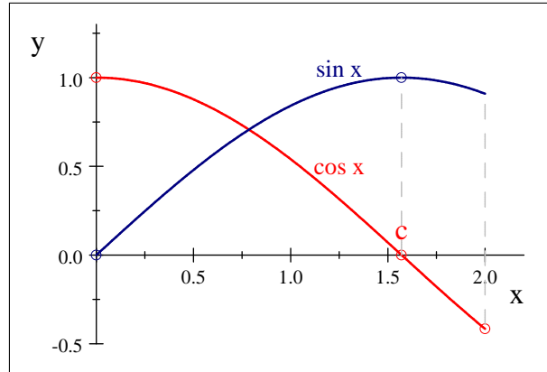
Die Graphen von Funktionen \cos x und \sin x auf dem Intervall [0, 2]
