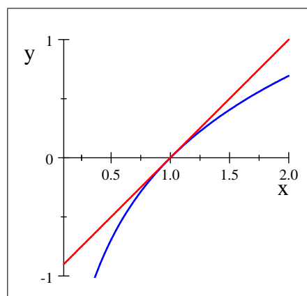
Die Funktionen \ln x (blau) und x - 1 (rot)
