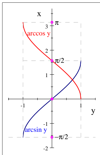
Funktionen arcsin und arccos
