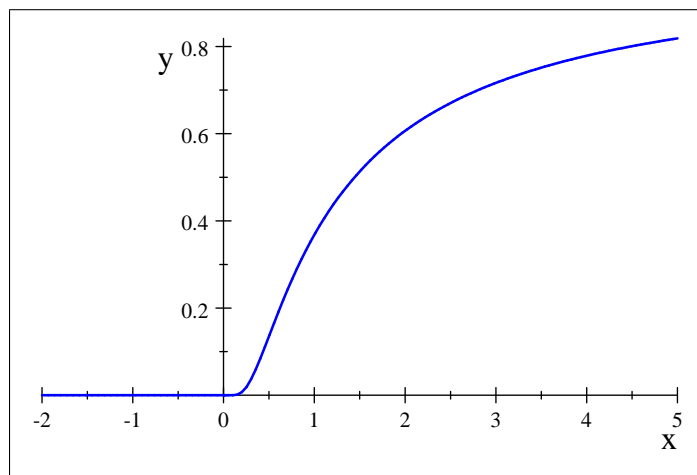
Der Graph der Funktion (7.16)
