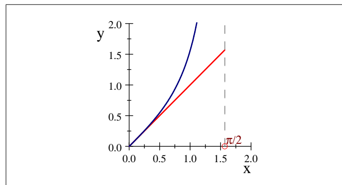
Die Graphen von Funktionen \tan x (blau) und x (rot)
