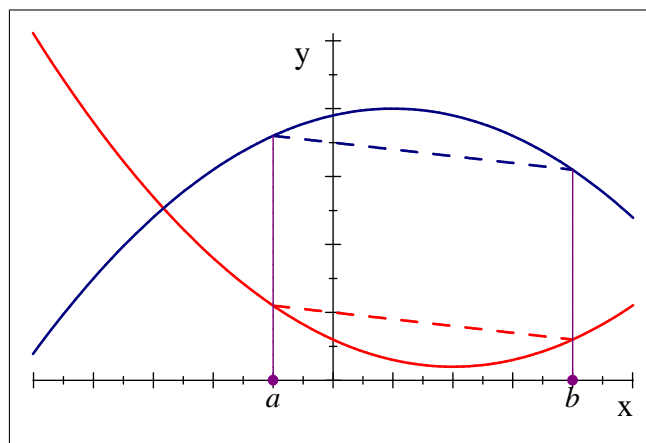
konvex - rot, konkav - blau
