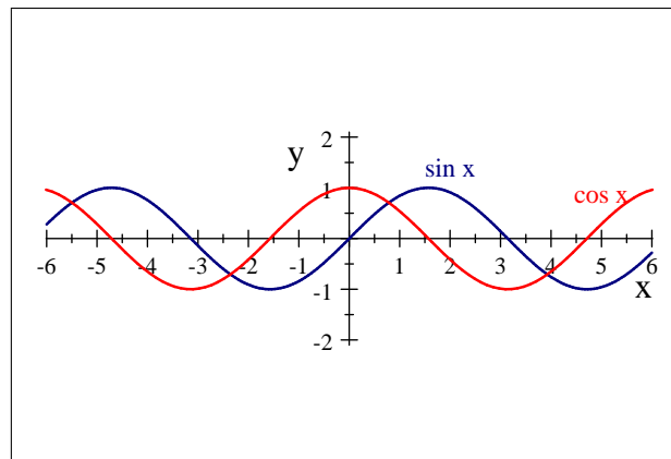
Die Graphen von Funktionen \cos x und \sin x
