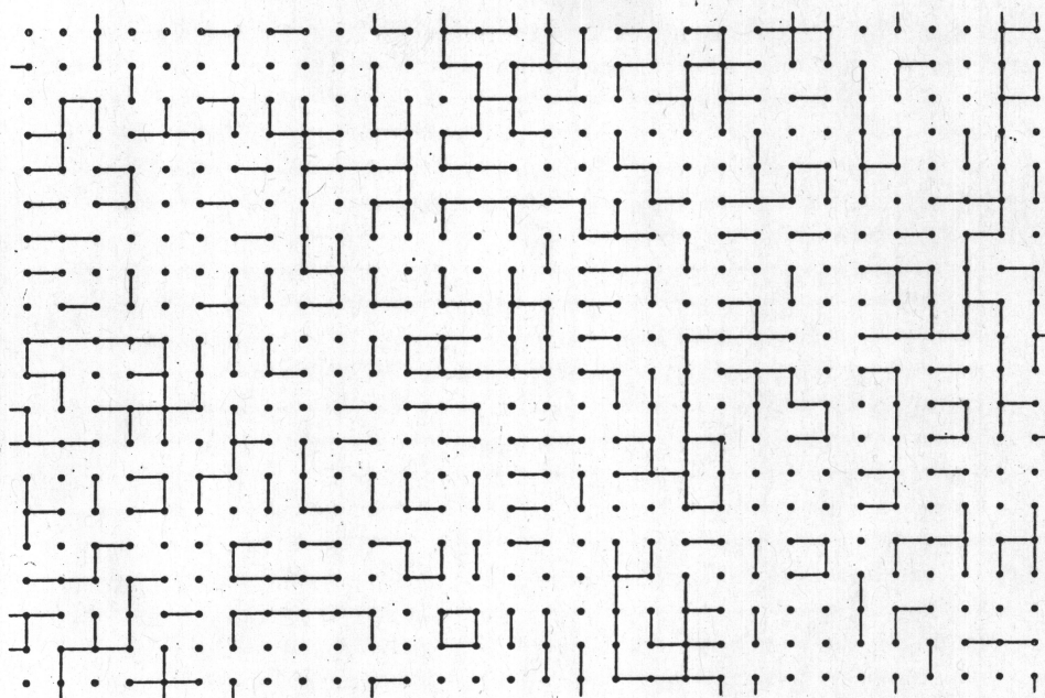
. Eine Kantenperkolaton auf dem Gitter \mathbb{Z}^2 mit p = 0,3 .
