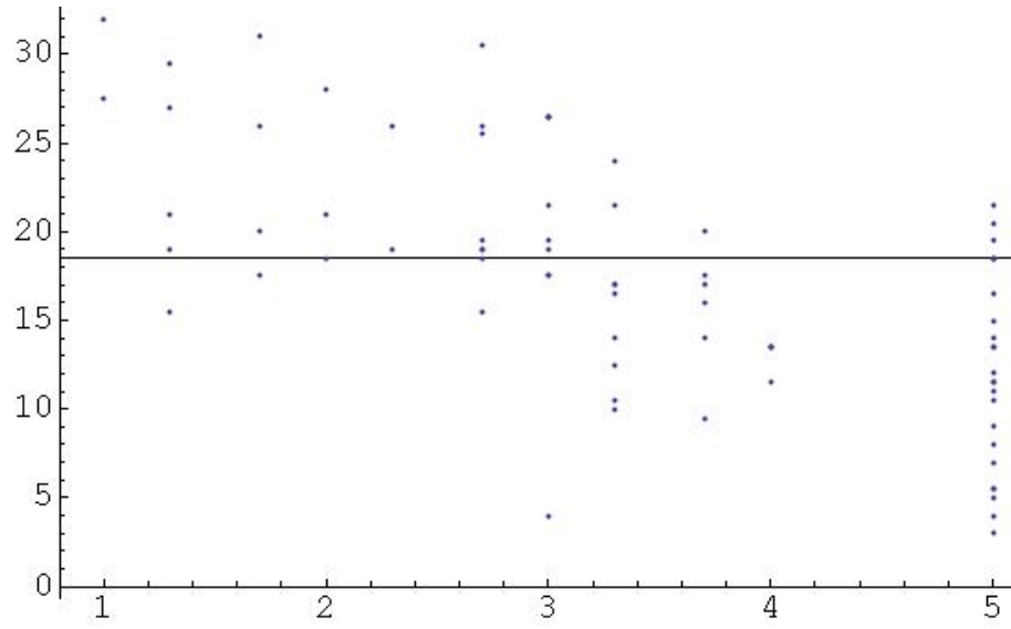
Abbildung 1: Auf der x -Achse die Noten der Klausur aus dem ersten Semester und auf der y -Achse die Punkteanzahl der Klausur aus dem zweiten Semester.
